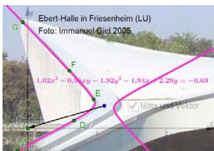
Abb. 5: Dachform als Hyperbel
